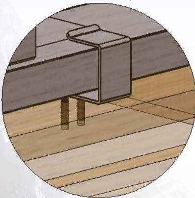
DETAIL B 1 : 2
